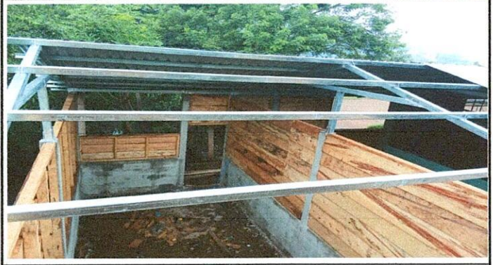
Foto 2: Instalación de estructuras metálicas y cubiertas de lamina.
